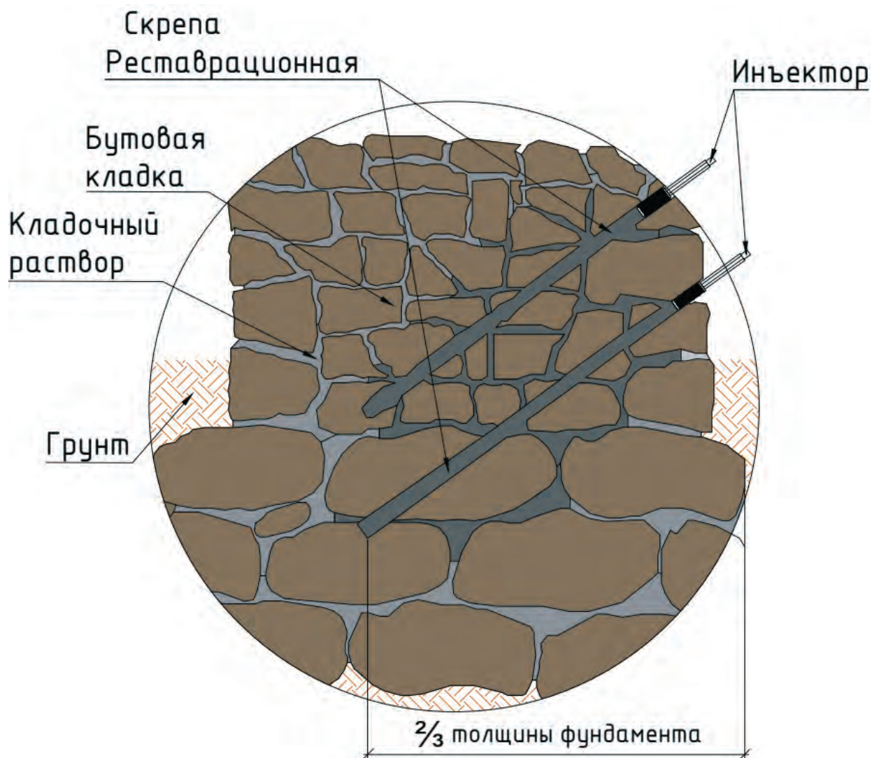
Рисунок А.4 – Схема реставрации каменной кладки
