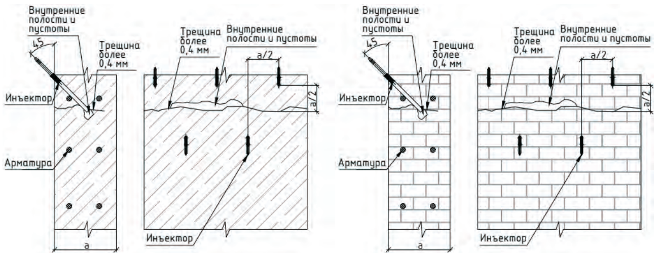
а) Фрагмент бетонной стены до ремонта, схема монтажа инъекторов
