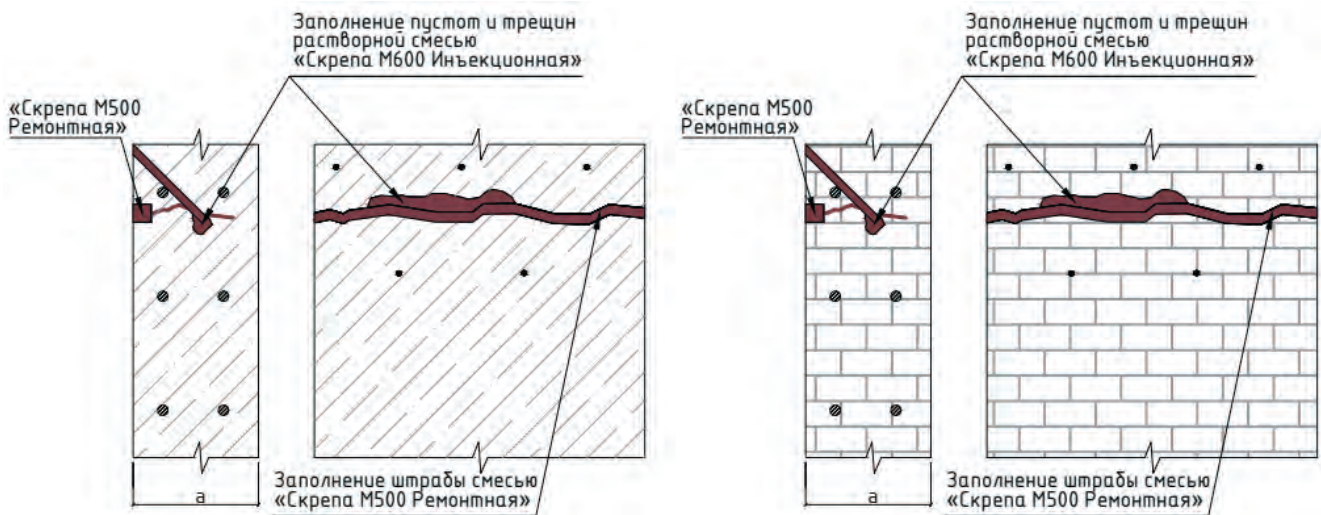
в) Фрагмент бетонной стены после ремонта
