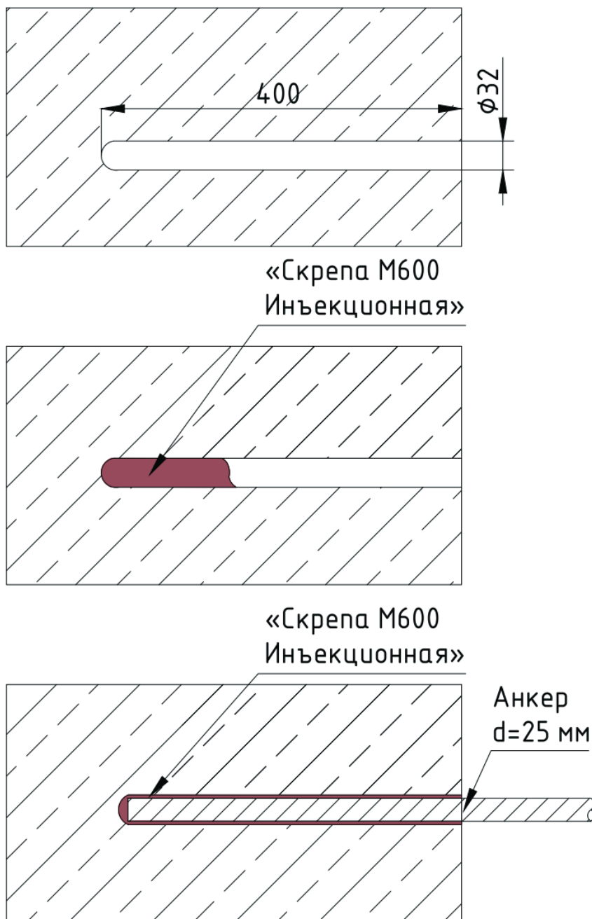
Рисунок А.5 – Схема закрепления анкера в строительной конструкции
